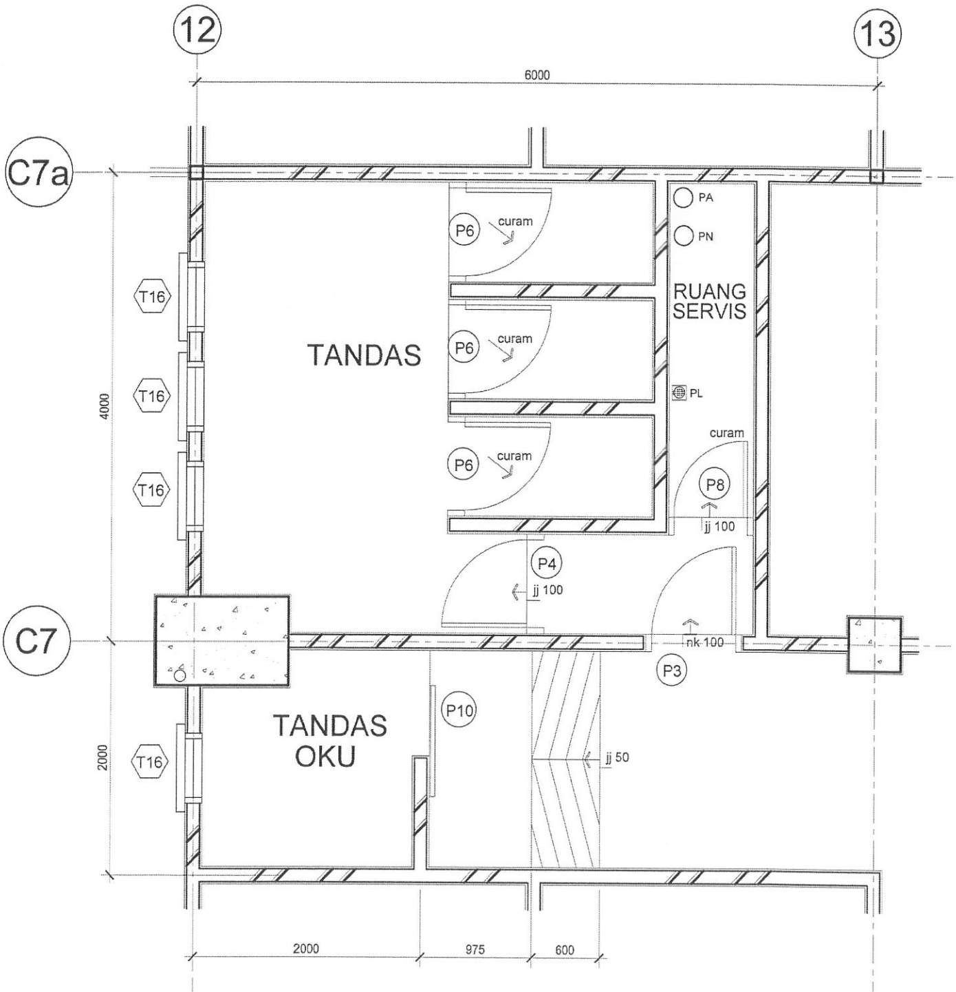
Pelan Lantai Tandas
