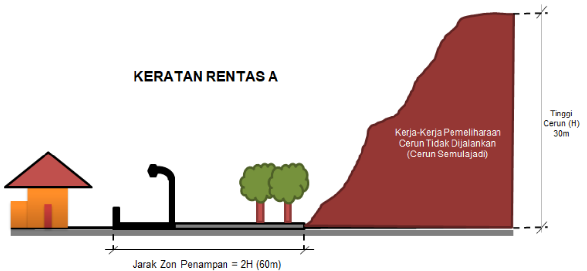
Rajah 2: Zon Penampam Minimum Bagi Cerun Potong atau Cerun Semulajadi Tanpa Pembaikan Cerun
