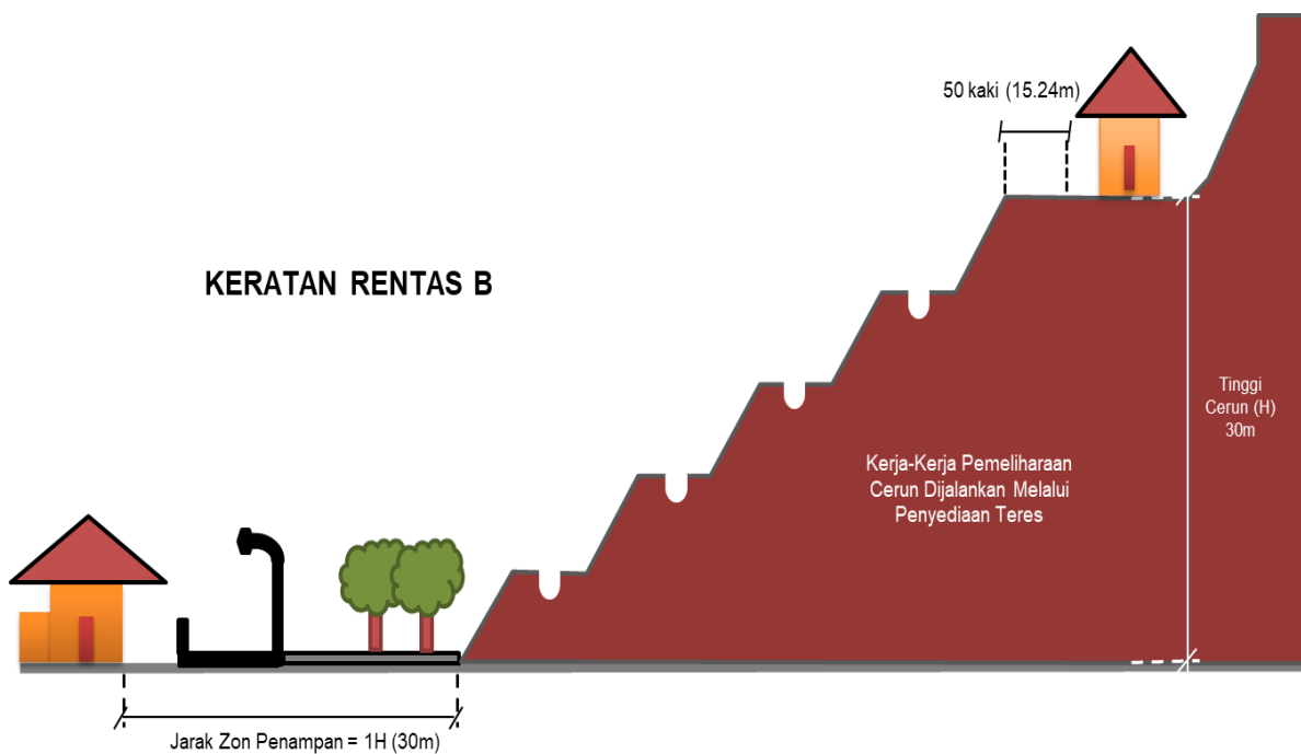
Rajah 3: Zon Penampam Minimum Bagi Cerun Potong atau Cerun Semulajadi Dengan Pembaikan Cerun
